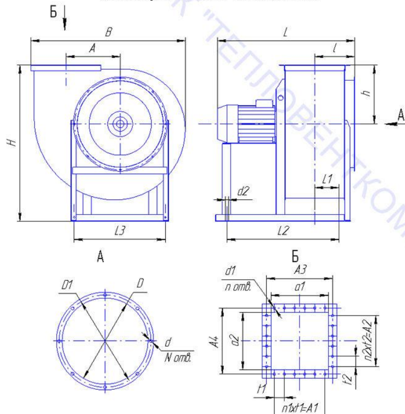
Вентилятор ВР 280-46 №2 – 8 1-е исполнение.
